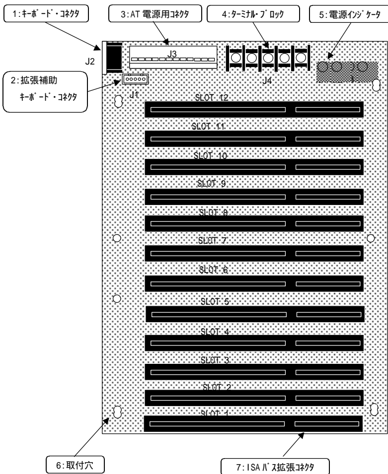
図 1 部品配置図
