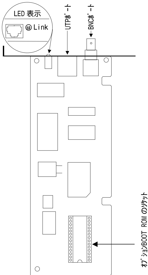
図 2・1 配置図
