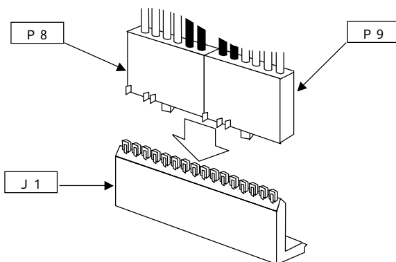
図 2 AT 電源コネクタの接続
