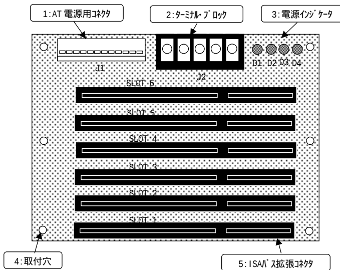
図 1 部品配置図
