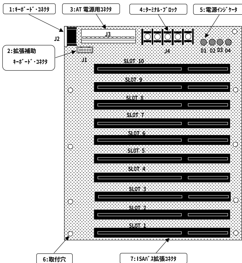
図 1 部品配置図
